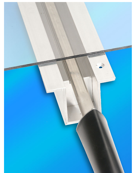
Heizstab flach - breite Erwärmung
